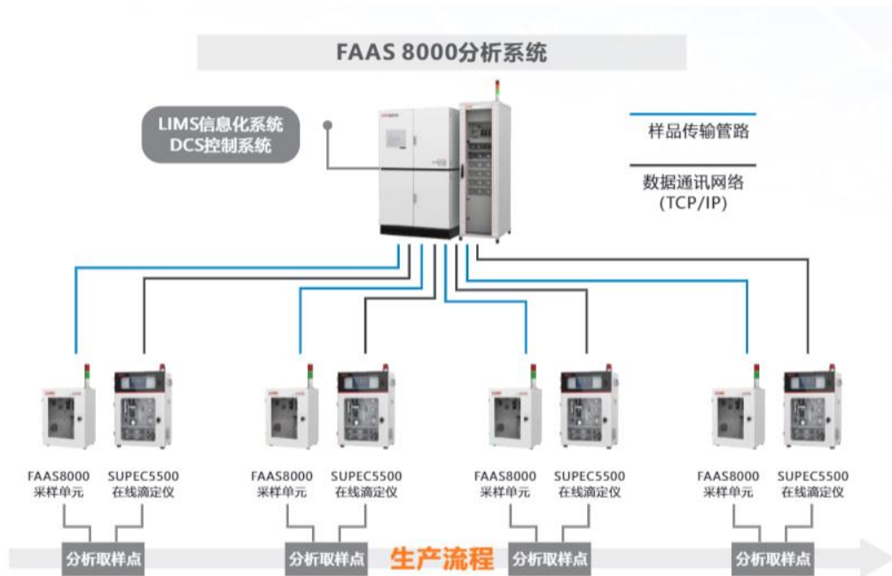
图10 工业过程成分智能在线分析系统
